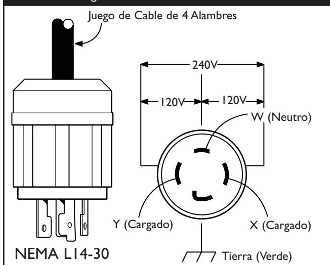
Figura 13 — 120/240 Volt AC, 30 Amperios, Receptáculo de Seguridad
